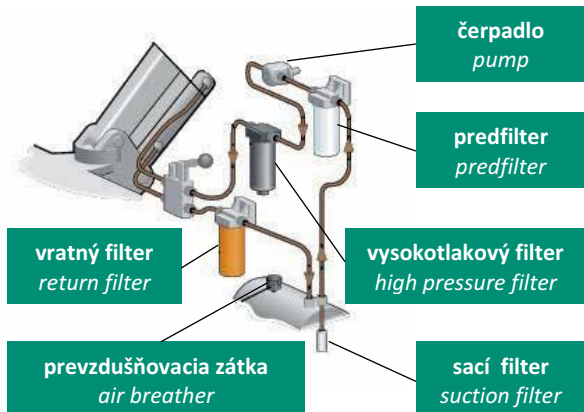
Typy olejových filtrov v hydraulickom okruhu: Types of oil filters in hydraulic circuit:
